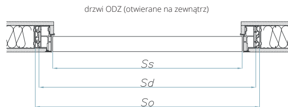
drzwi ODZ (otwierane na zewnątrz)
